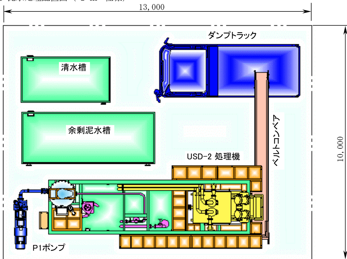
6-1 泥水処理配置図（2 m 3 仕様）
