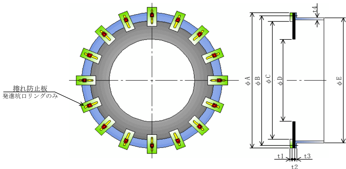
発進立坑用坑口リング
