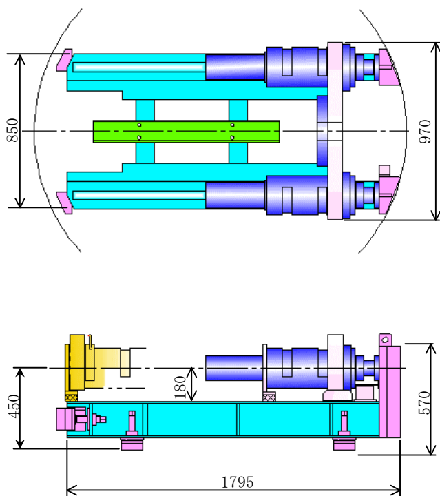
Fs-2 (φ 250～φ 300)
