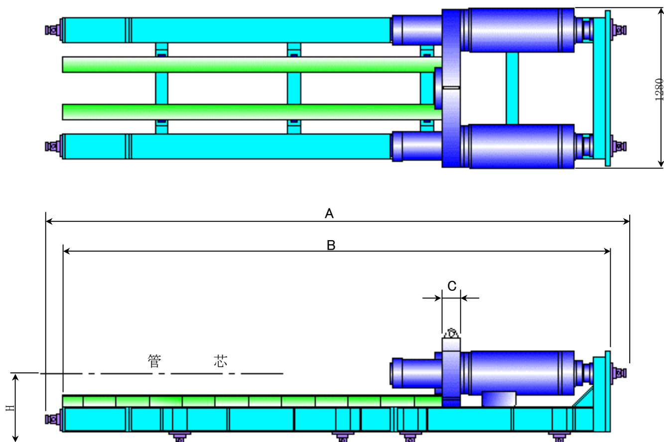
元押装置寸法表
