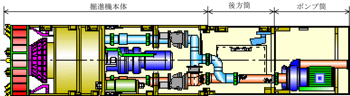
ポンプ筒接続図 (例：φ 700mm)
