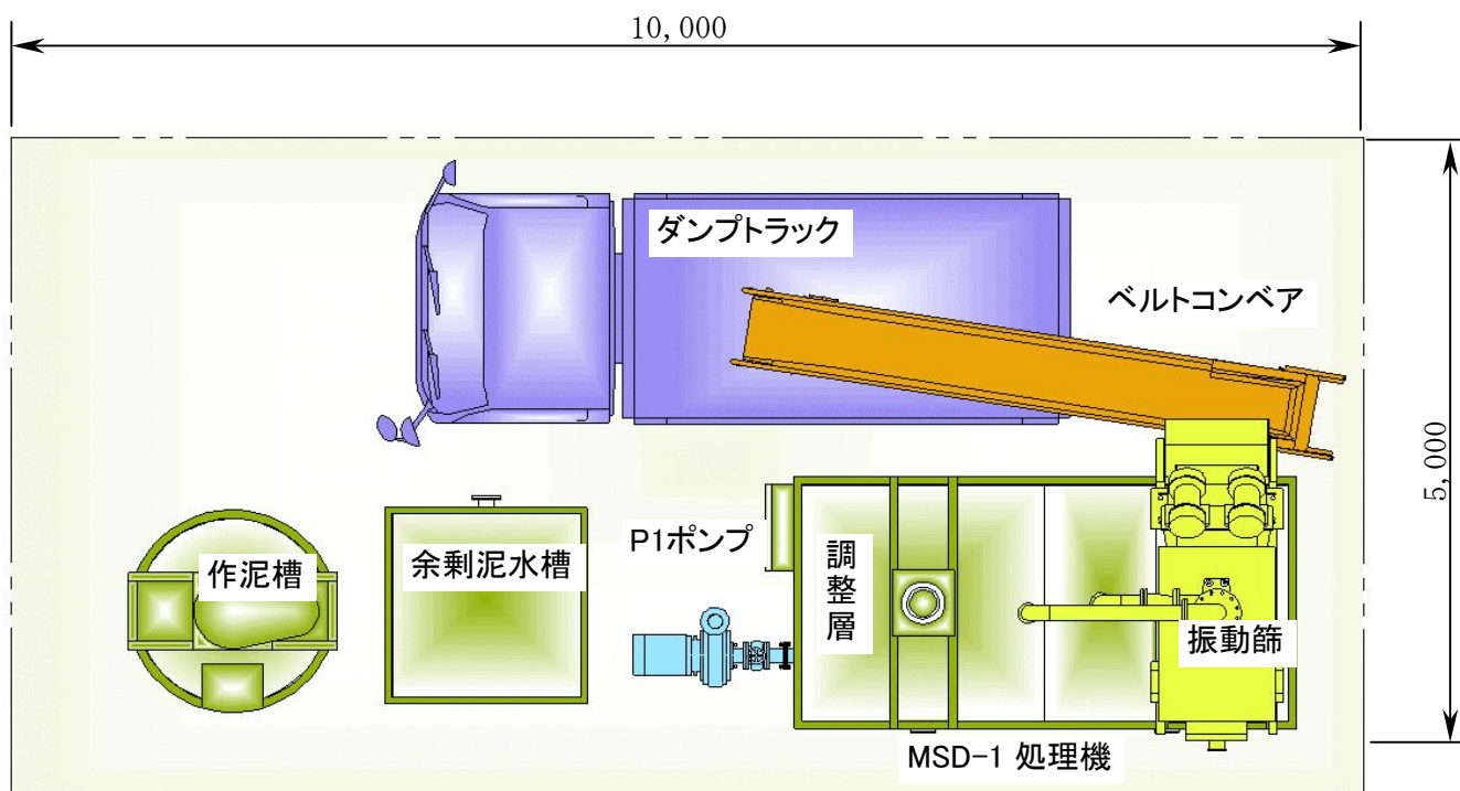
21-3-2 泥水処理配置図（1 m 3 仕様）
