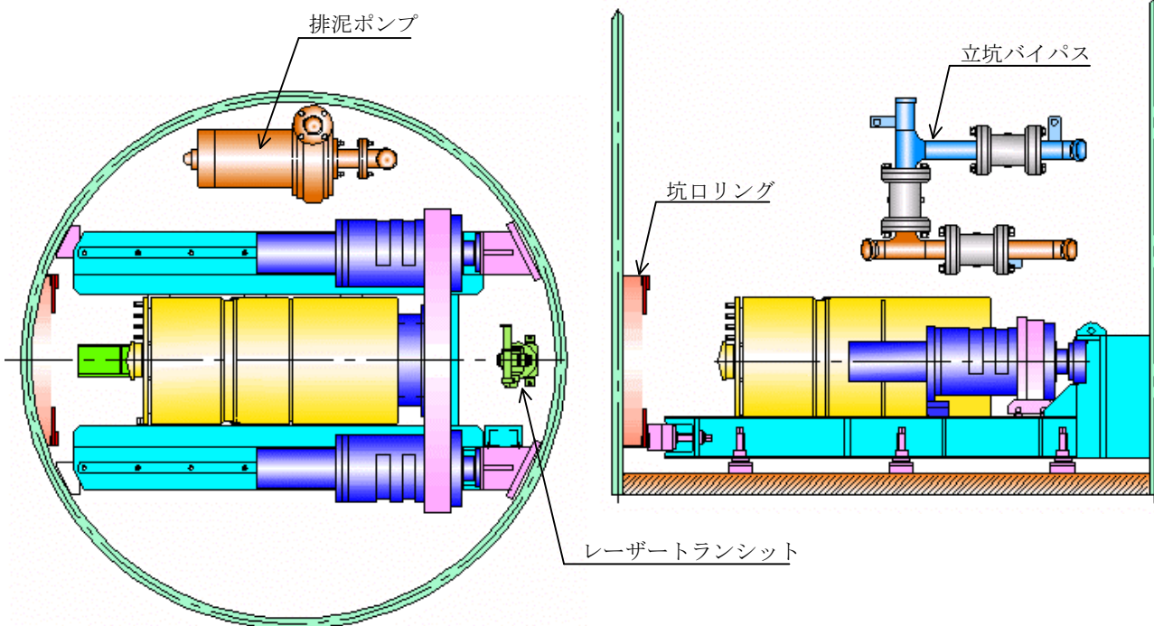
φ 2,500 発進立坑図
