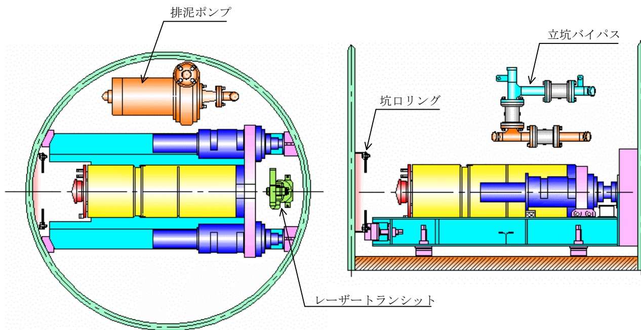
φ 2,500 発進立坑図
