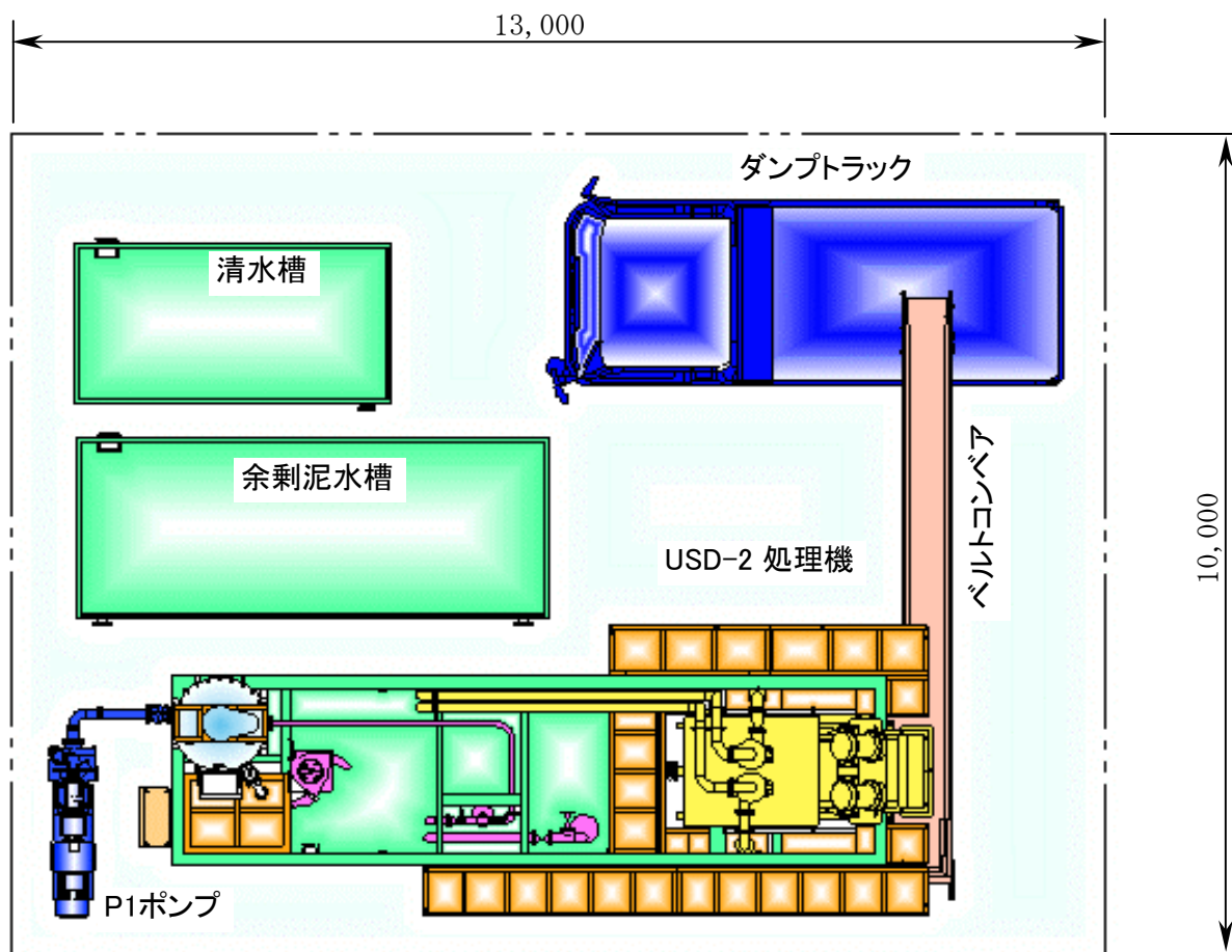
21-3-3 泥水処理配置図（2 m 3 仕様）
